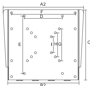
Soporte de LCD/Monitor
