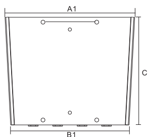
Soporte de pared
